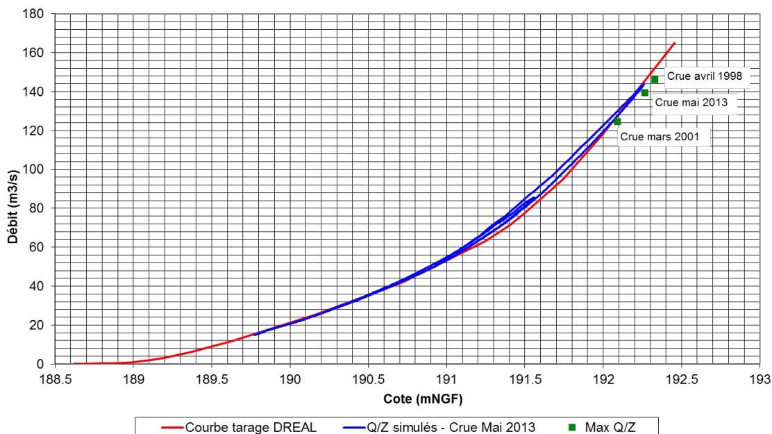
Courbe de tarage simulée à la station hydrométrique de Dissangis
